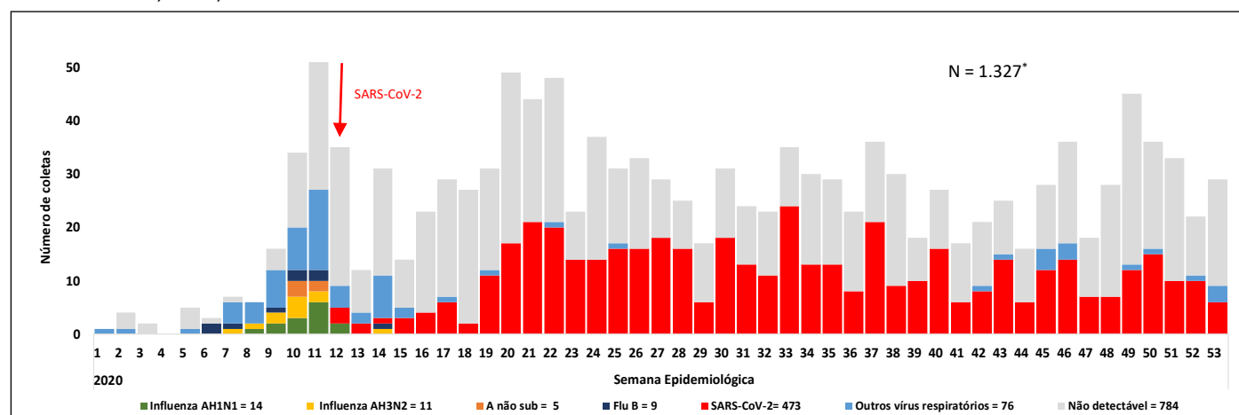
Figura 1. Frequência de amostras coletadas em unidades sentinelas, segundo semana epidemiológica do início dos sintomas. Distrito Federal, 2020, 2021 e 2022 até a SE 12.
