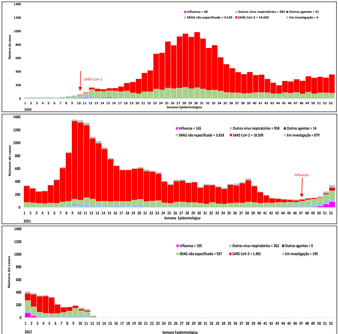
Figura 3. Distribuição dos casos de SRAG, segundo agente etiológico e semana epidemiológica do início dos sintomas, de residentes do Distrito Federal. Distrito Federal, 2020, 2021 e 2022 até a SE 12.
