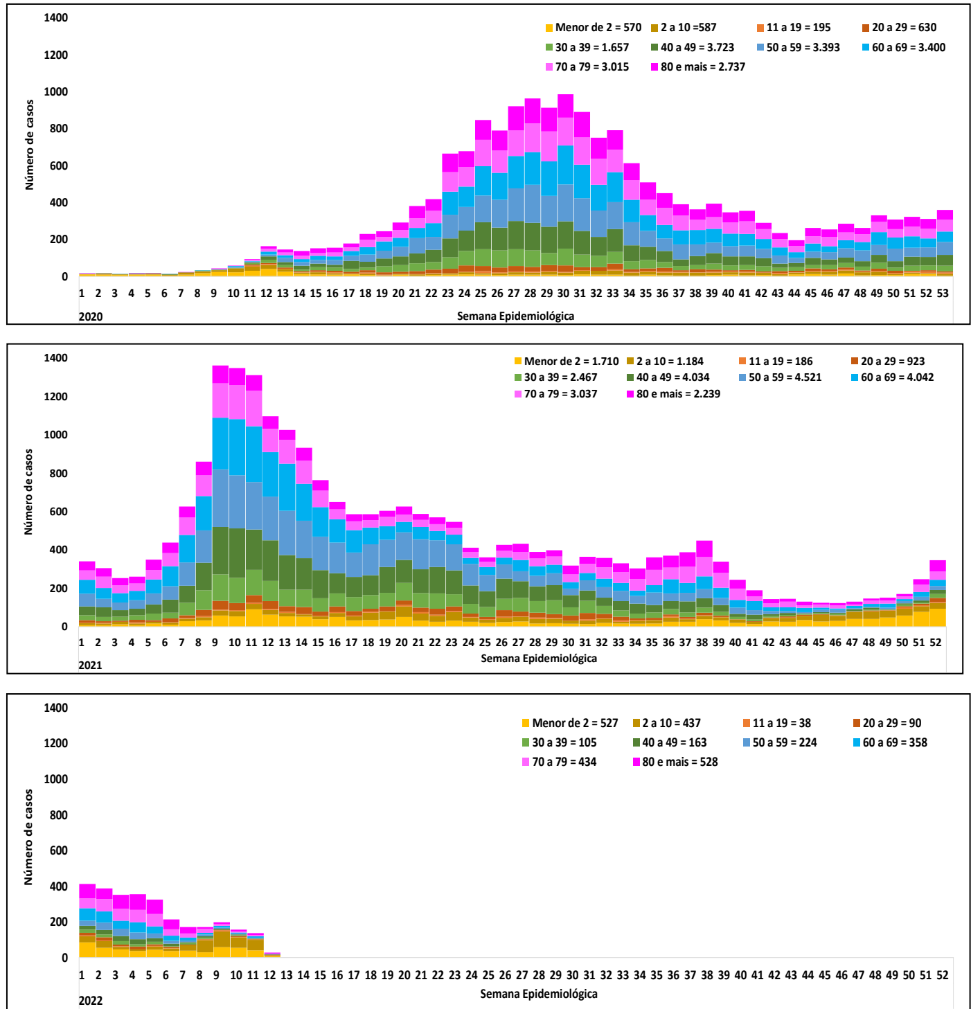
Figura 4. Distribuição dos casos de SRAG, segundo faixa etária e semana epidemiológica do início dos sintomas, de residentes do Distrito Federal. Distrito Federal, 2020, 2021 e 2022 até a SE 12.
