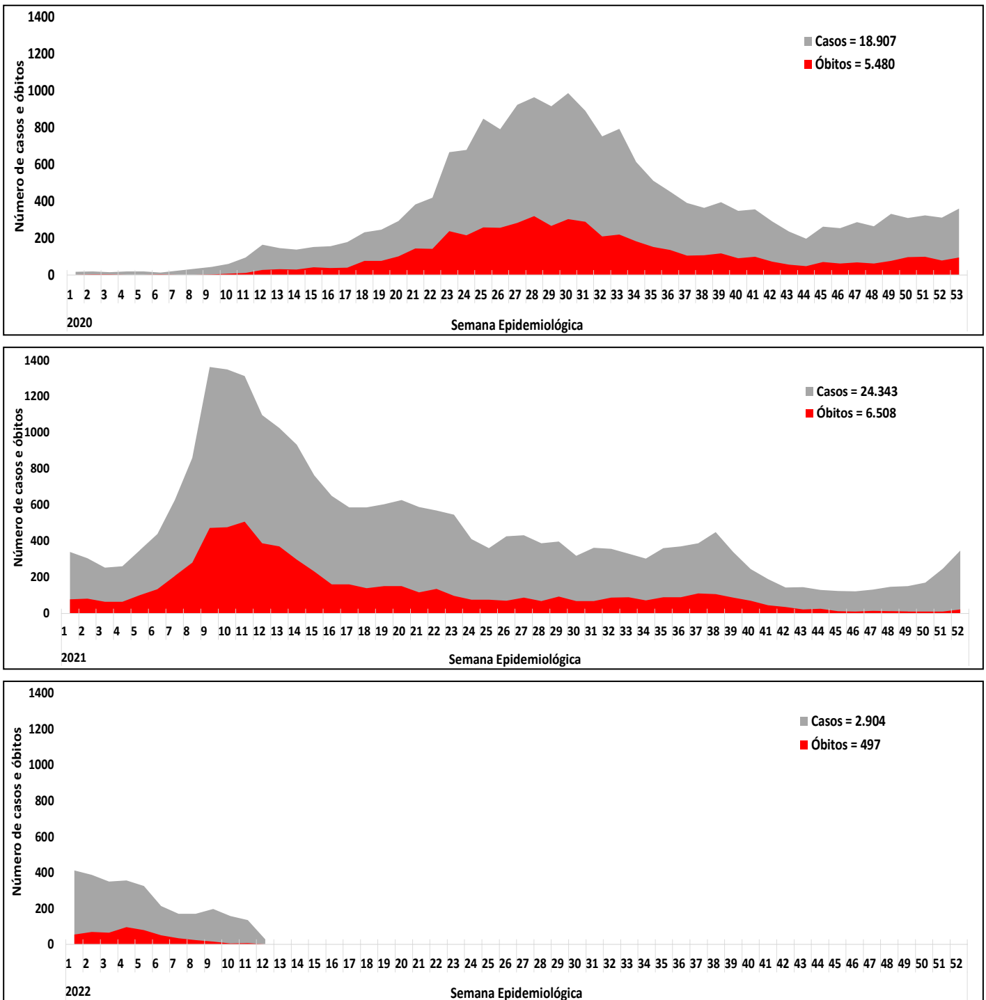
Figura 2. Distribuição dos casos e óbitos de SRAG, segundo semana epidemiológica do início dos sintomas, de residentes do Distrito Federal, 2020, 2021 e 2022 até a SE 12.
