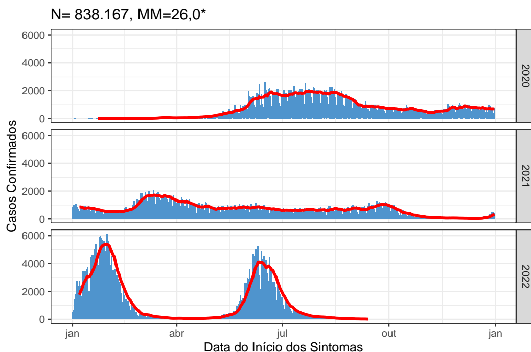
Figura 4: Média móvel dos casos confirmados no Distrito Federal, 13 de setembro de 2022
