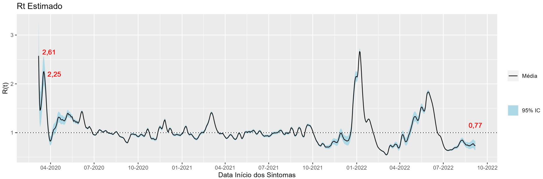
Figura 6: R(t) estimado para os dados oficiais de infectados por Covid-19 no DF segundo a data de início dos sintomas dos casos no Distrito Federal, 13 de setembro de 2022
