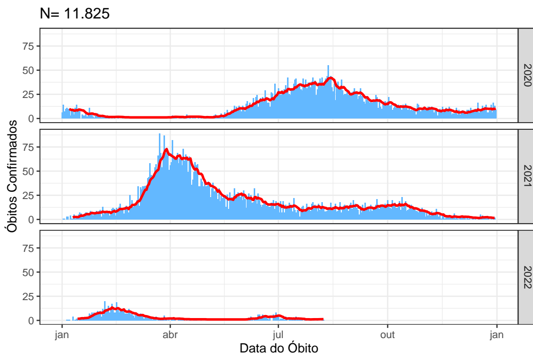
Figura 5: Média móvel dos óbitos confirmados no Distrito Federal, 13 de setembro de 2022
