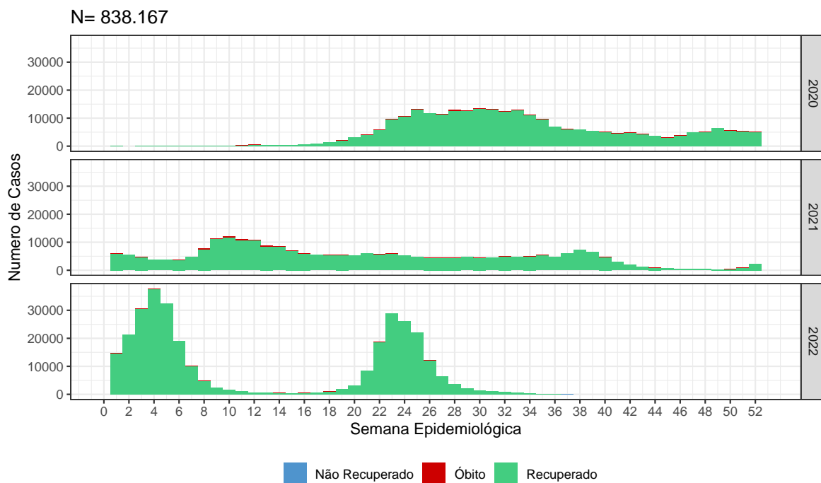
Figura 1: Curva epidemiológica de casos confirmados de COVID-19 segundo evolução e data de início de sintomas, Distrito Federal, 13 de setembro de 2022
