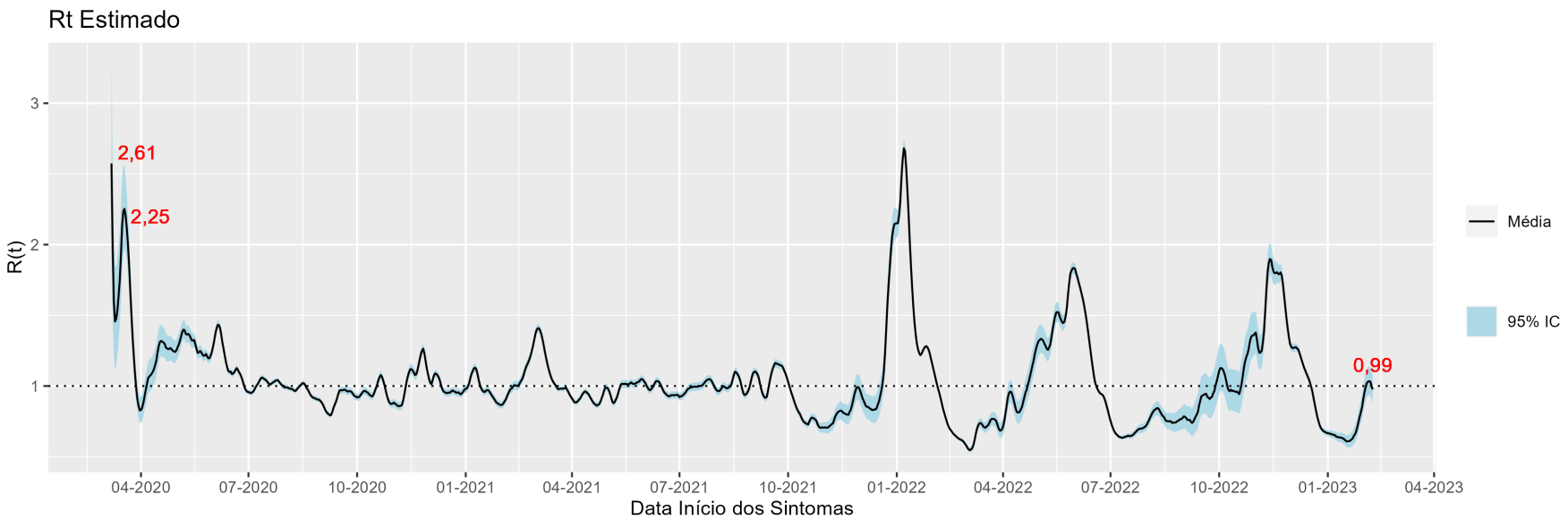
Figura 6: R(t) estimado para os dados oficiais de infectados por Covid-19 no DF segundo a data de início dos sintomas dos casos no Distrito Federal, 15 de fevereiro de 2023
