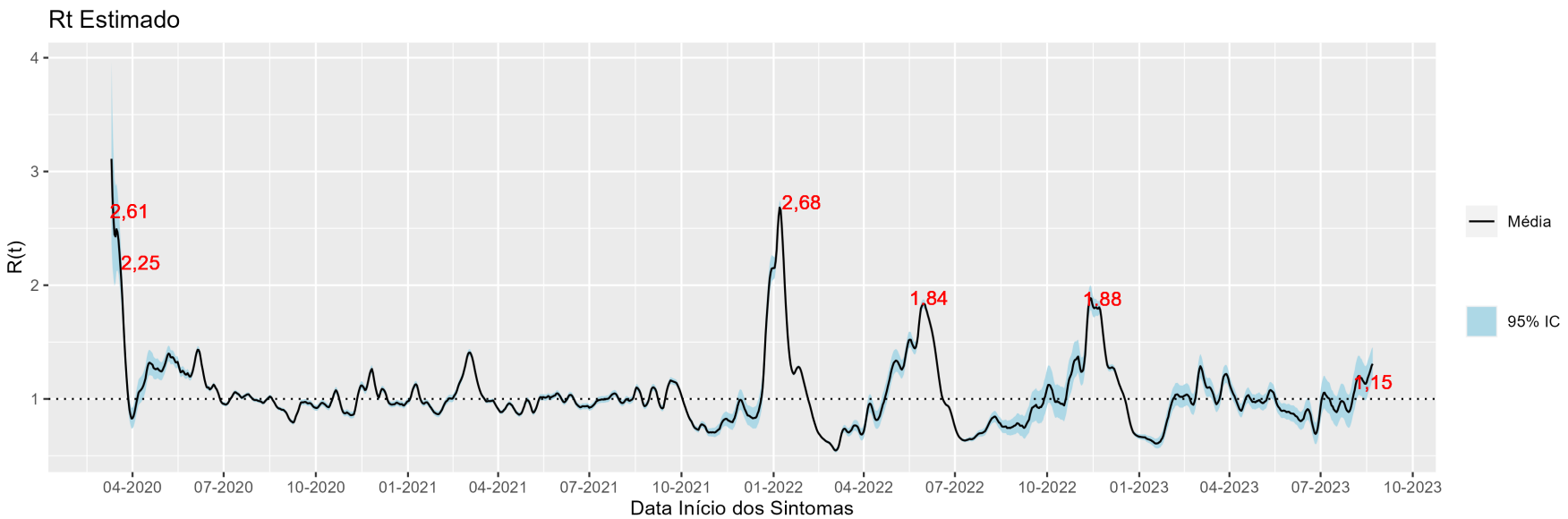
Figura 6: R(t) estimado para os dados oficiais de infectados por Covid-19 no DF segundo a data de início dos sintomas dos casos no Distrito Federal, 29 de agosto de 2023
