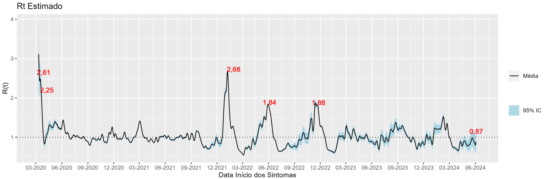
Figura 6: R(t) estimado para os dados oficiais de infectados por Covid-19 no DF segundo a data de início dos sintomas dos casos no Distrito Federal, 11 de junho de 2024
