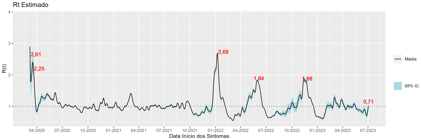
Figura 6: R(t) estimado para os dados oficiais de infectados por Covid-19 no DF segundo a data de início dos sintomas dos casos no Distrito Federal, 10 de julho de 2023
