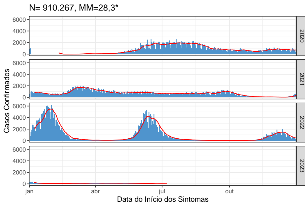
Figura 4: Média móvel dos casos confirmados no Distrito Federal, 10 de julho de 2023
