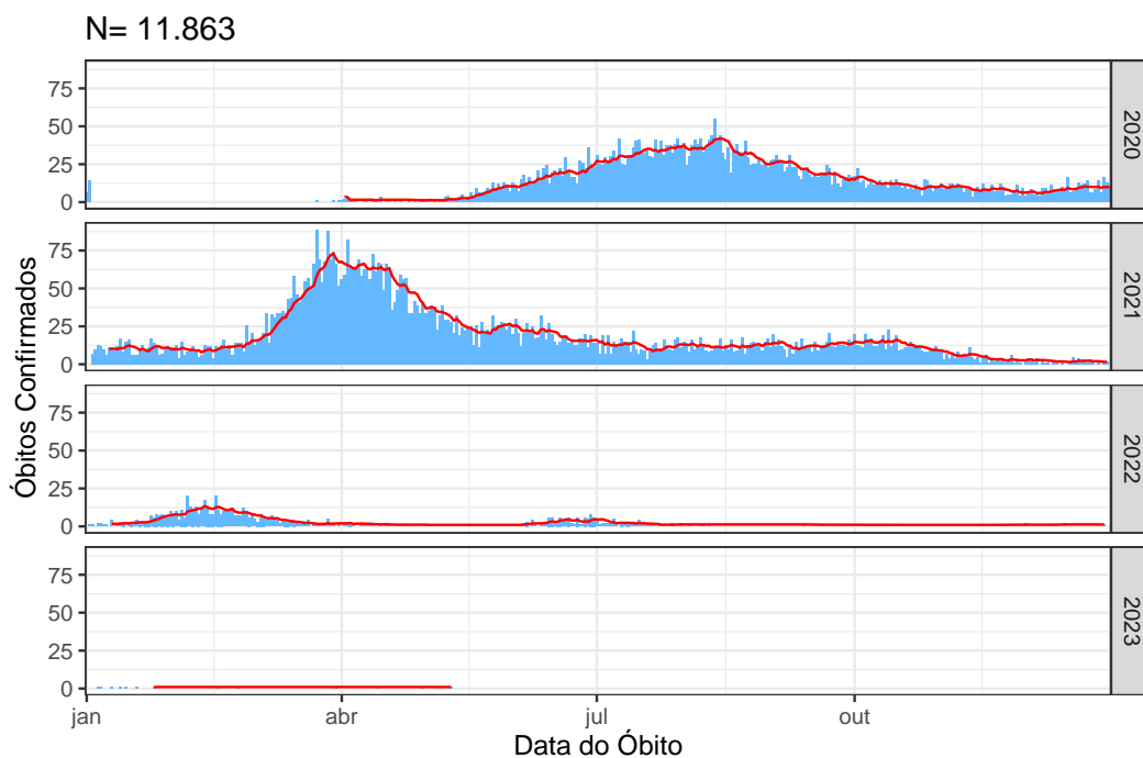
Figura 5: Média móvel dos óbitos confirmados no Distrito Federal, 10 de julho de 2023
