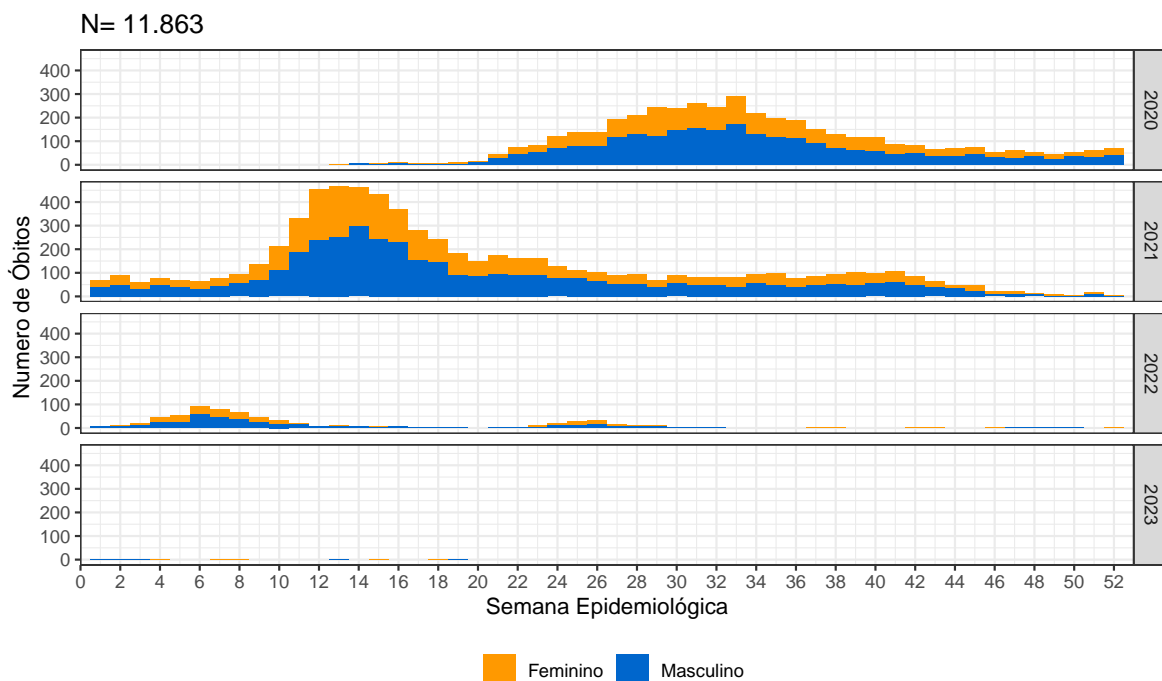
Figura 2: Curva de óbitos confirmados de COVID-19 segundo evolução e data de início de sintomas, Distrito Federal, 10 de julho de 2023
