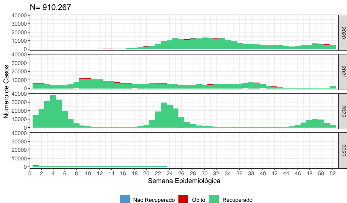
Figura 1: Curva epidemiológica de casos confirmados de COVID-19 segundo evolução e data de início de sintomas, Distrito Federal, 10 de julho de 2023
