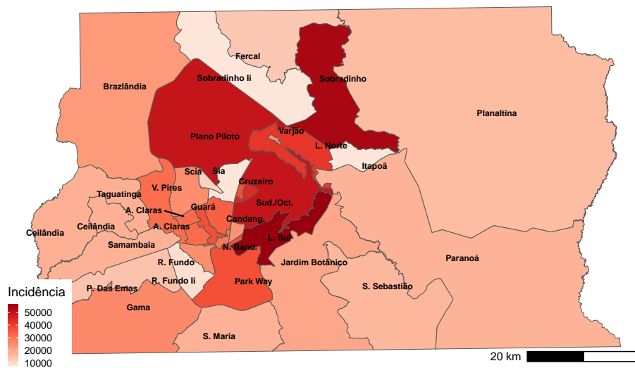
Figura 3: Distribuição geográfica de incidência de casos por 100 mil habitantes, segundo Região Administrativa. Distrito Federal, 10 de julho de 2023
