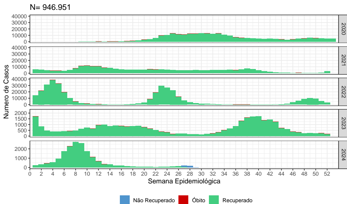
Figura 1: Curva epidemiológica de casos confirmados de COVID-19 segundo evolução e data de início de sintomas, Distrito Federal, 16 de julho de 2024
