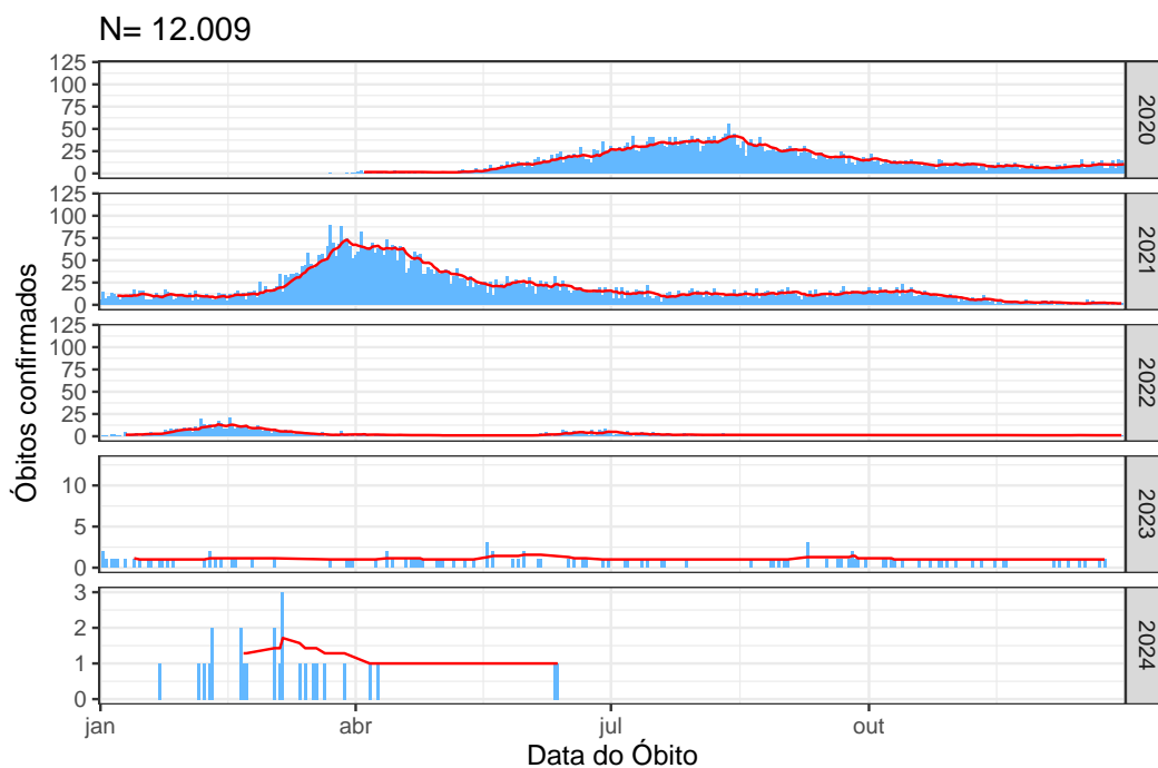
Figura 5: Média móvel dos óbitos confirmados no Distrito Federal, 16 de julho de 2024
