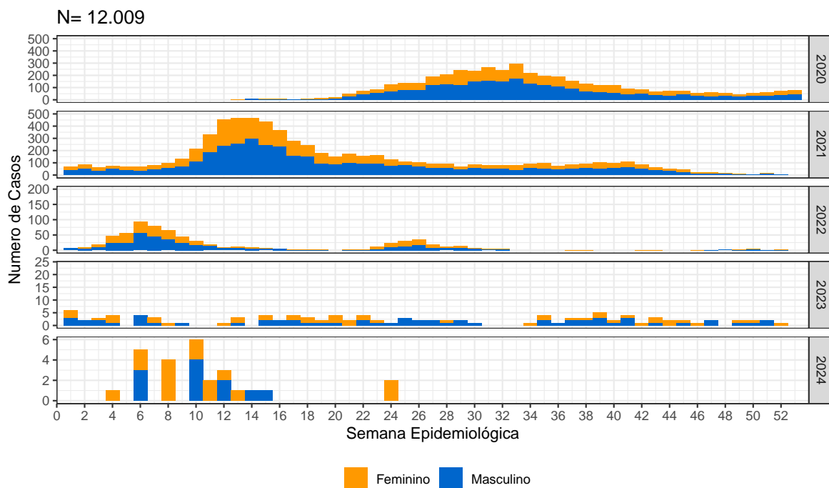
Figura 2: Curva de óbitos confirmados de COVID-19 segundo evolução e data de início de sintomas, Distrito Federal, 16 de julho de 2024
