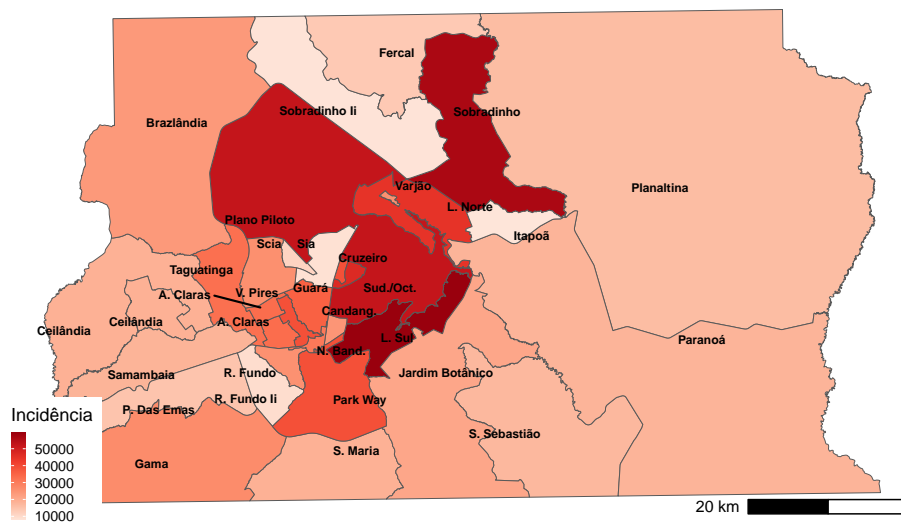
Figura 3: Distribuição geográfica de incidência de casos por 100 mil habitantes, segundo Região Administrativa. Distrito Federal, 16 de julho de 2024
