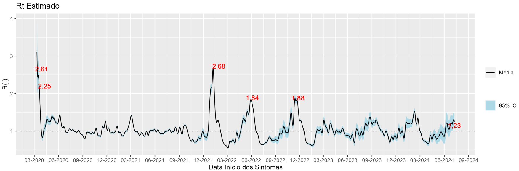
Figura 6: R(t) estimado para os dados oficiais de infectados por Covid-19 no DF segundo a data de início dos sintomas dos casos no Distrito Federal, 16 de julho de 2024
