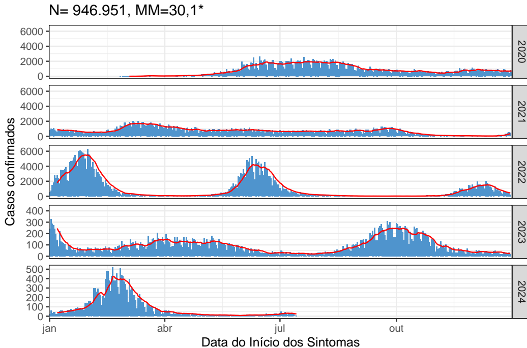
Figura 4: Média móvel dos casos confirmados no Distrito Federal, 16 de julho de 2024
