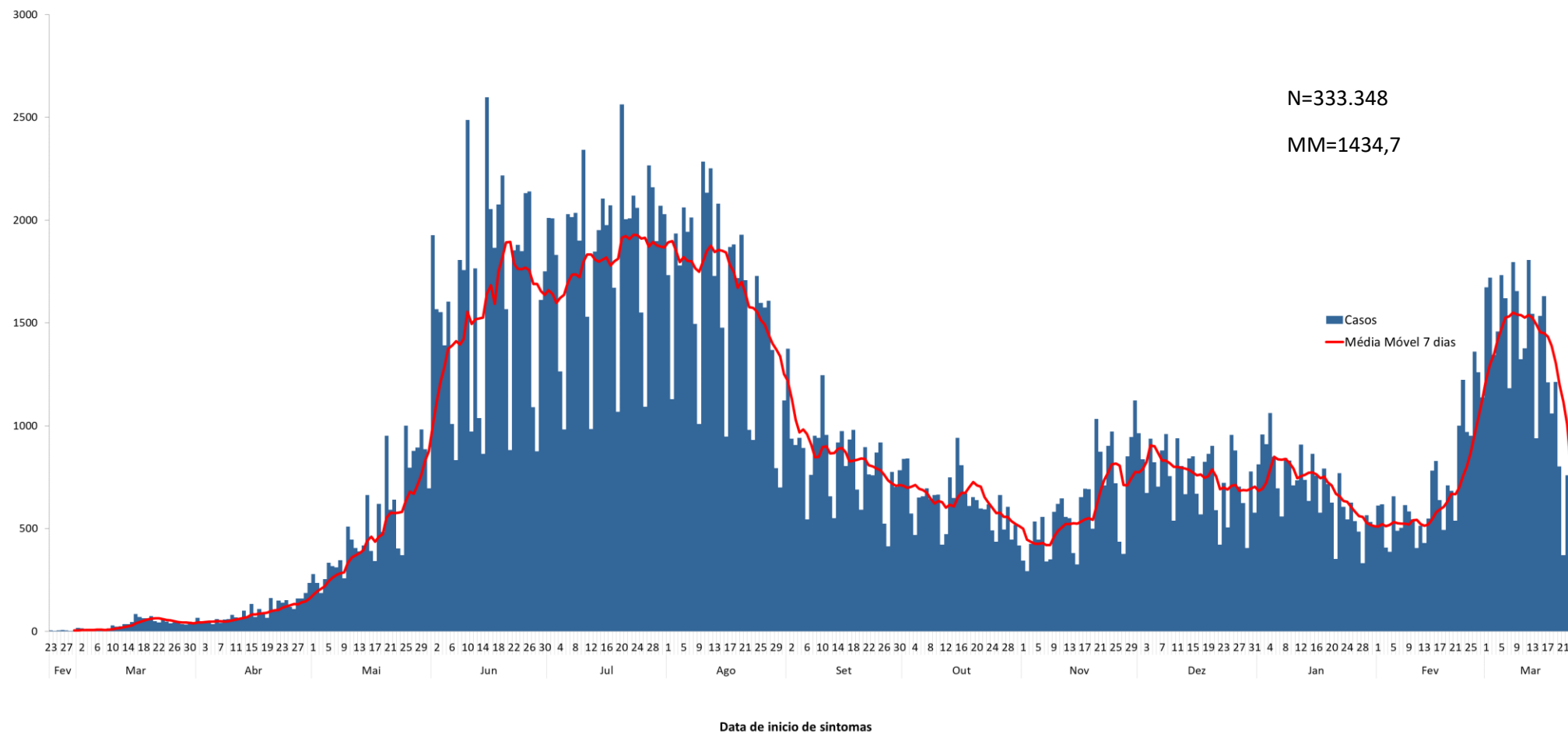
Figura 4. Média móvel dos casos confirmados no Distrito Federal, 24 de março de 2021.
