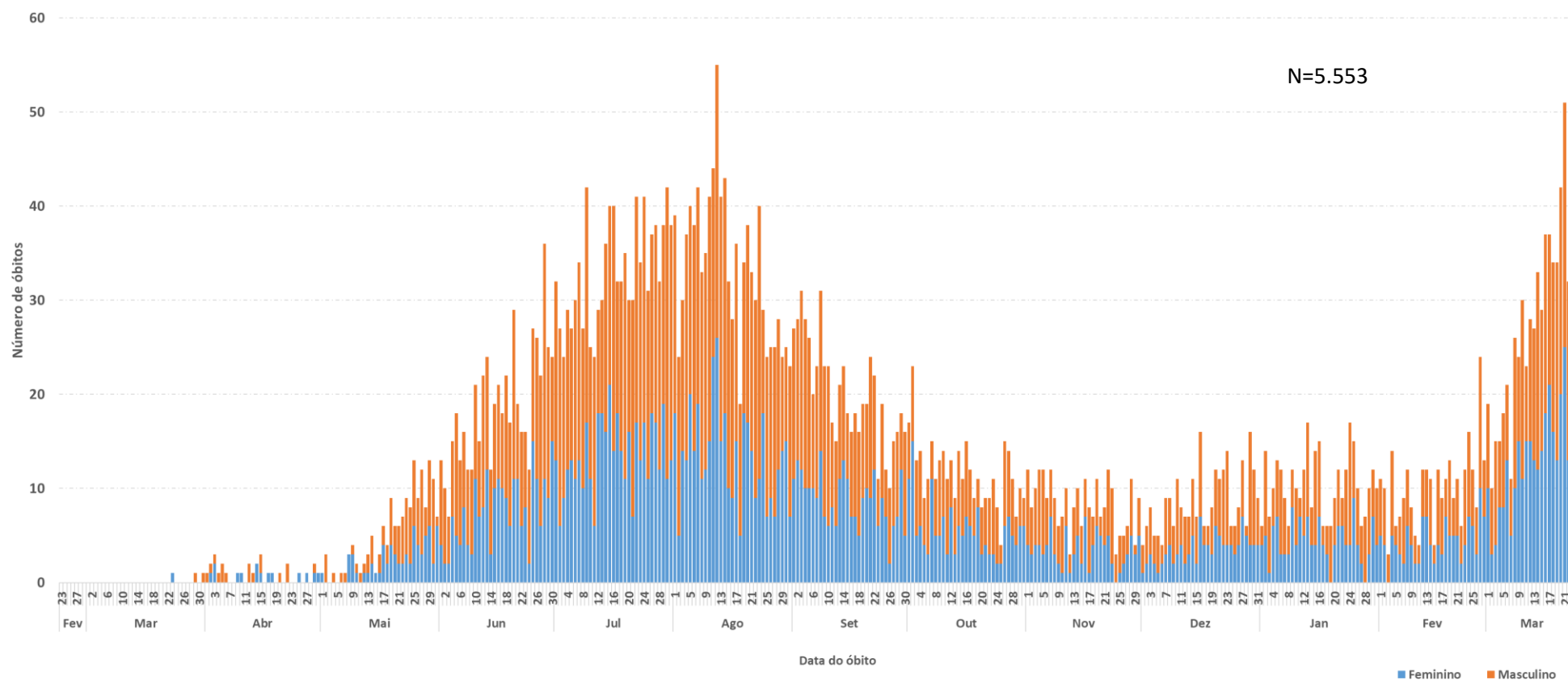
Figura 2. Curva dos óbitos confirmados de COVID-19 notificados no DF, segundo a data de ocorrência do óbito, 24 de março de 2021.
