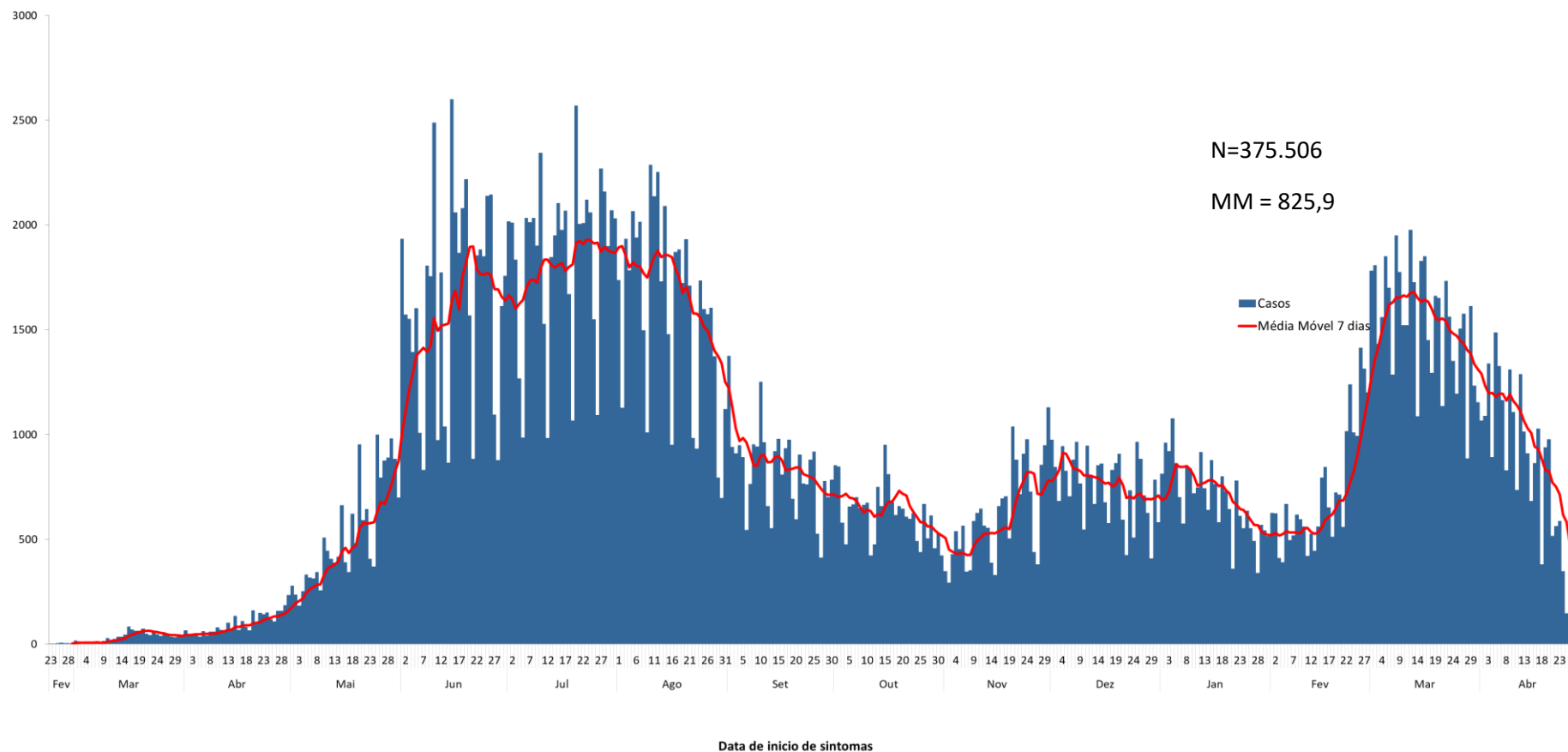
Figura 4. Média móvel dos casos confirmados no Distrito Federal, 27 de abril de 2021.
