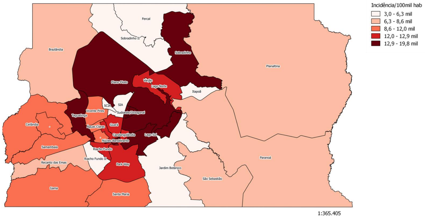
Figura 3. Distribuição geográfica de incidência de casos por 100 mil habitantes, segundo Região Administrativa. Distrito Federal, 27 de abril de 2021.
