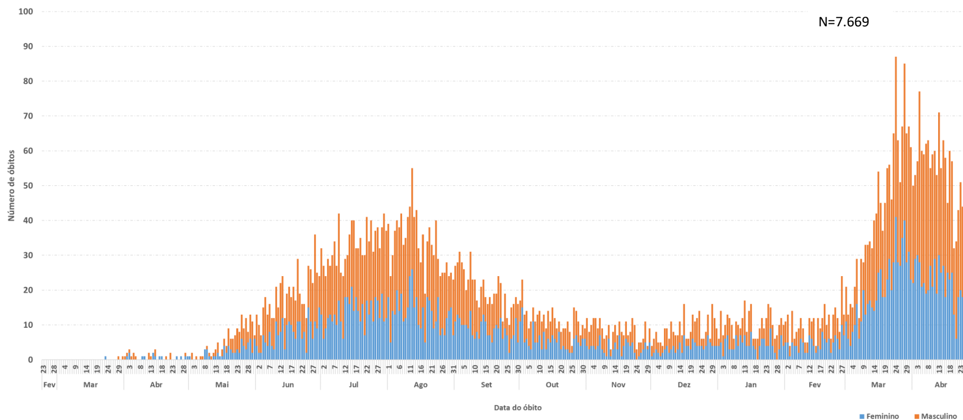
Figura 2. Curva dos óbitos confirmados de COVID-19 notificados no DF, segundo a data de ocorrência do óbito, 27 de abril de 2021.
