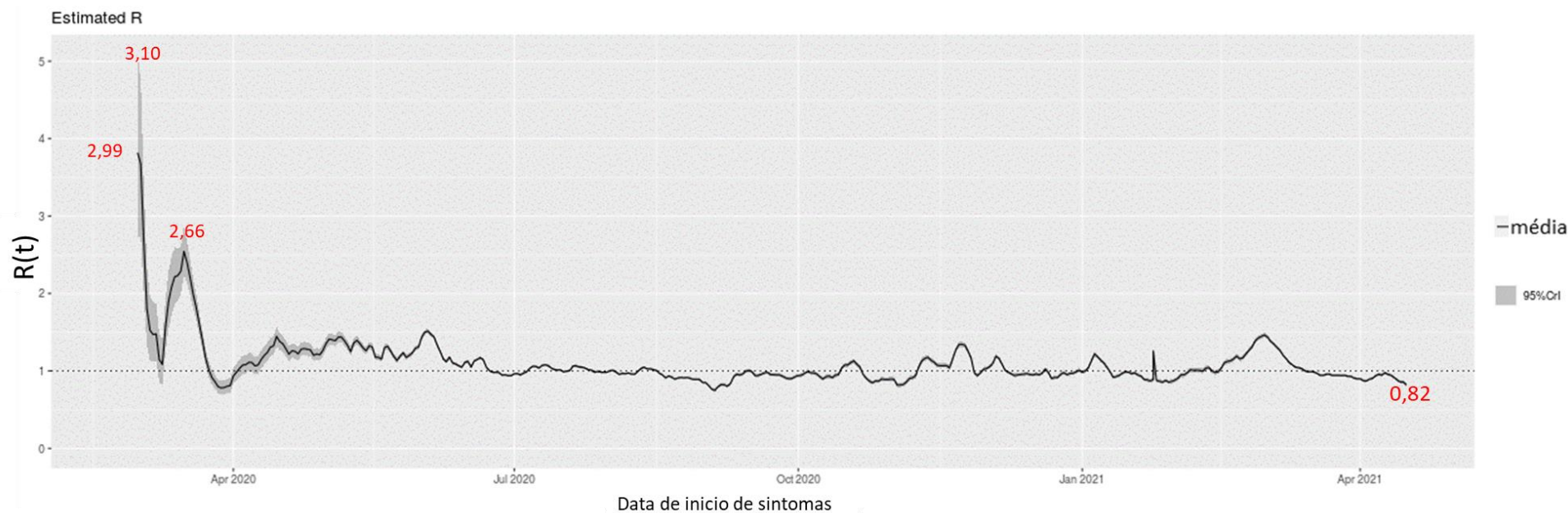
Figura 6. R(t) estimado para os dados oficiais de infectados por Covid-19 no DF segundo a data de início dos sintomas dos casos no Distrito Federal, 27 de abril de 2021.
