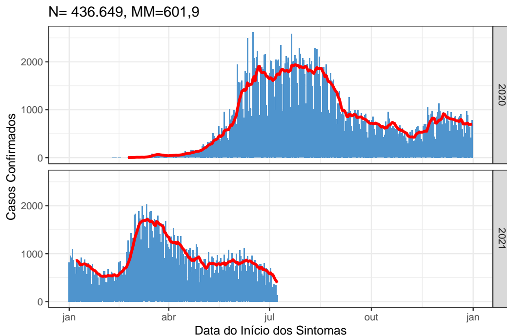
Figura 4: Média móvel dos casos confirmados no Distrito Federal, 09 de julho de 2021
