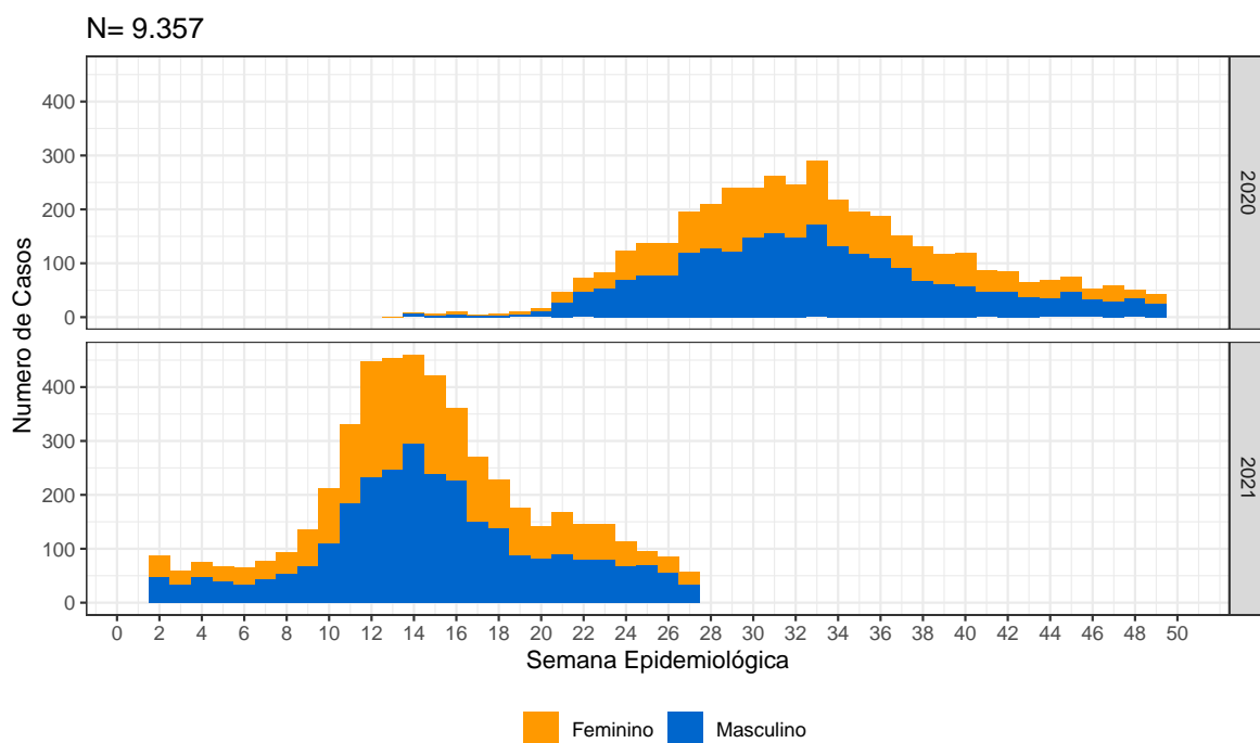
Figura 2: Curva de óbitos confirmados de COVID-19 segundo evolução e data de início de sintomas, Distrito Federal, 09 de julho de 2021
