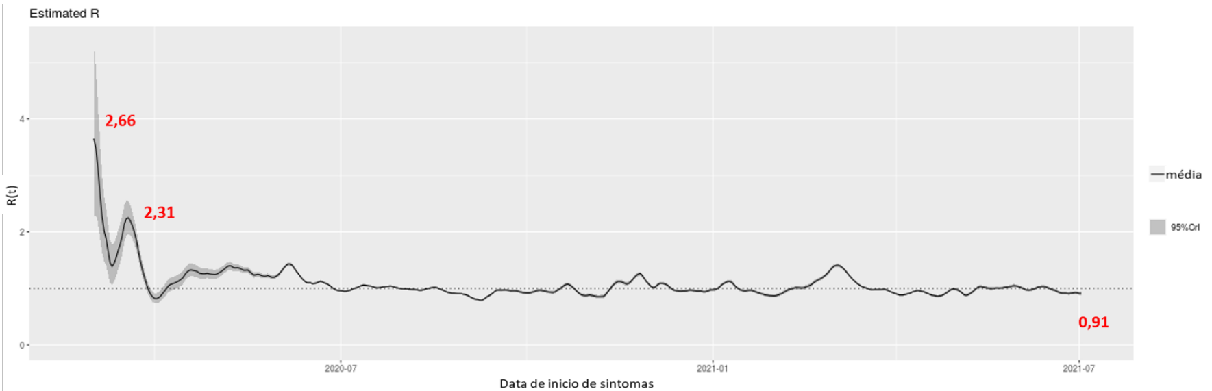
Figura 6: R(t) estimado para os dados oficiais de infectados por Covid-19 no DF segundo a data de início dos sintomas dos casos no Distrito Federal, 09 de julho de 2021
