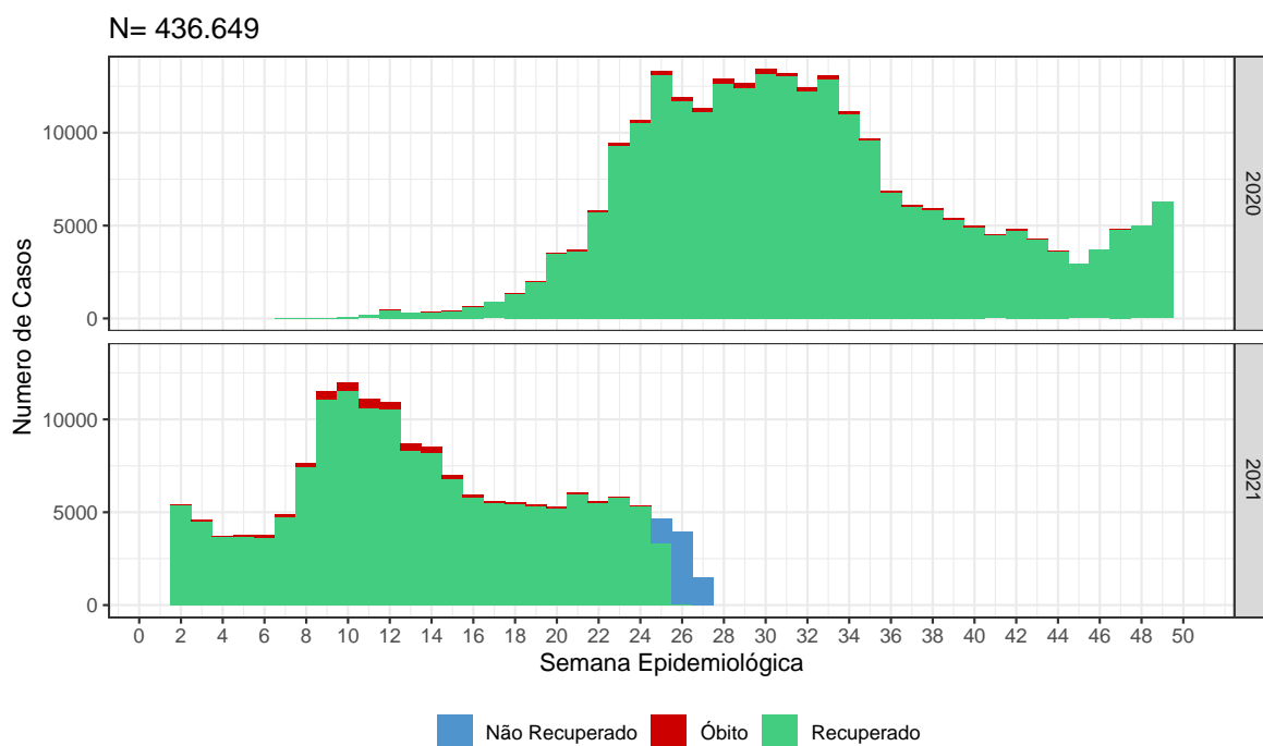
Figura 1: Curva epidemiológica de casos confirmados de COVID-19 segundo evolução e data de início de sintomas, Distrito Federal, 09 de julho de 2021
