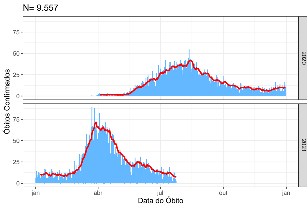
Figura 5: Média móvel dos óbitos confirmados no Distrito Federal, 25 de julho de 2021
