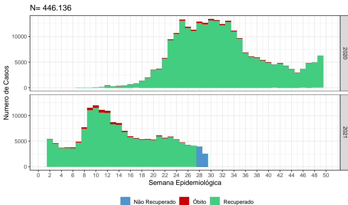
Figura 1: Curva epidemiológica de casos confirmados de COVID-19 segundo evolução e data de início de sintomas, Distrito Federal, 25 de julho de 2021
