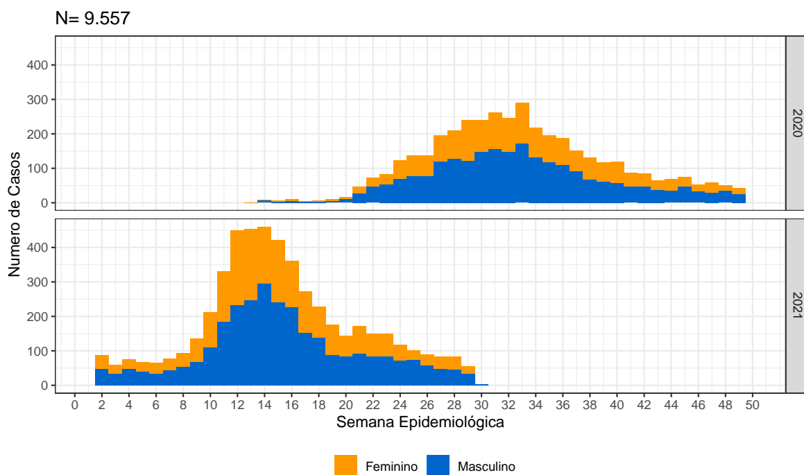
Figura 2: Curva de óbitos confirmados de COVID-19 segundo evolução e data de início de sintomas, Distrito Federal, 25 de julho de 2021
