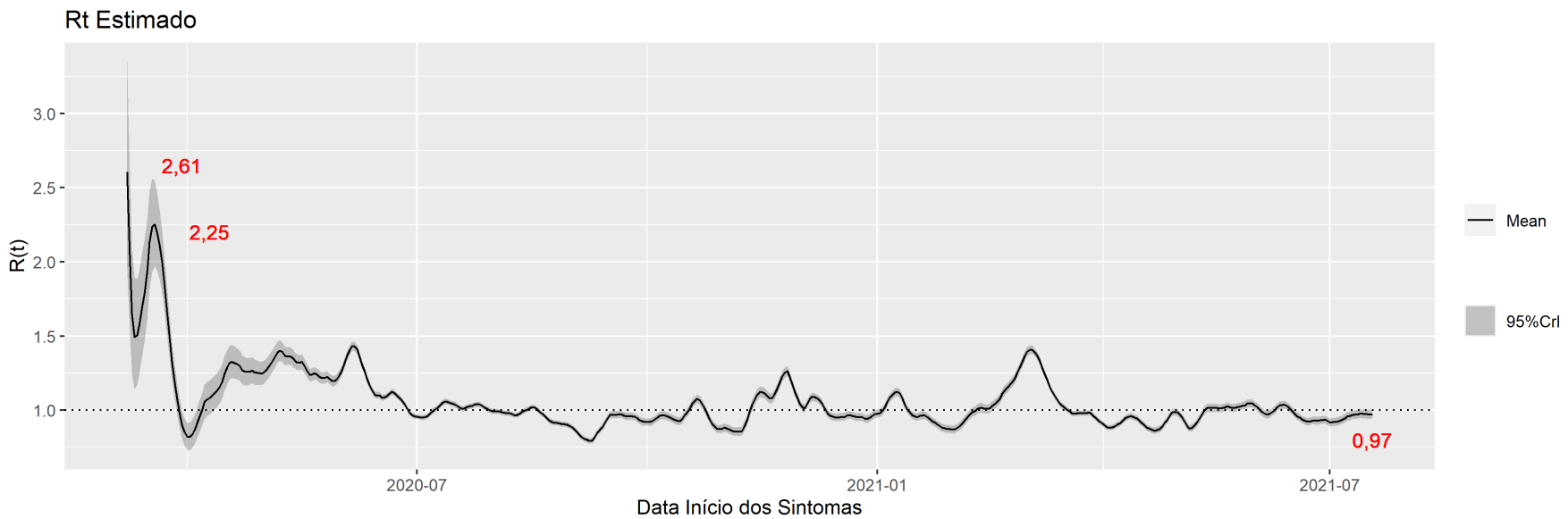
Figura 6: R(t) estimado para os dados oficiais de infectados por Covid-19 no DF segundo a data de início dos sintomas dos casos no Distrito Federal, 25 de julho de 2021
