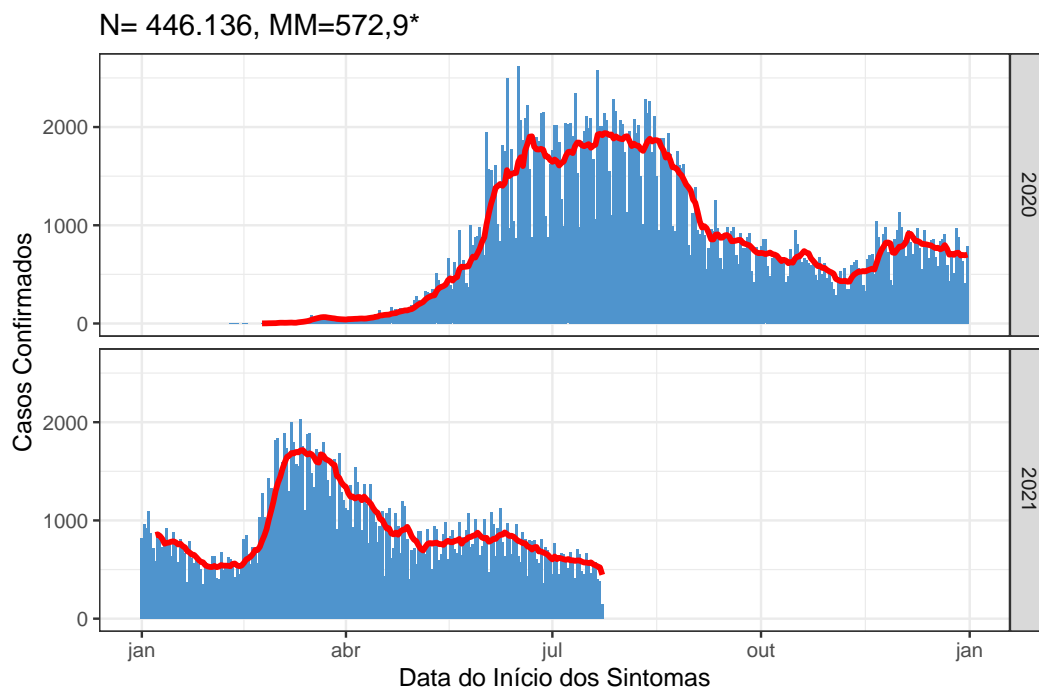
Figura 4: Média móvel dos casos confirmados no Distrito Federal, 25 de julho de 2021
