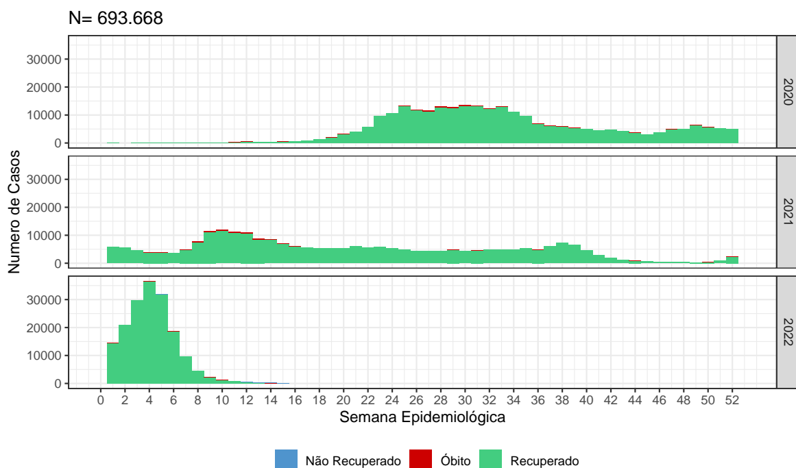
Figura 1: Curva epidemiológica de casos confirmados de COVID-19 segundo evolução e data de início de sintomas, Distrito Federal, 11 de abril de 2022
