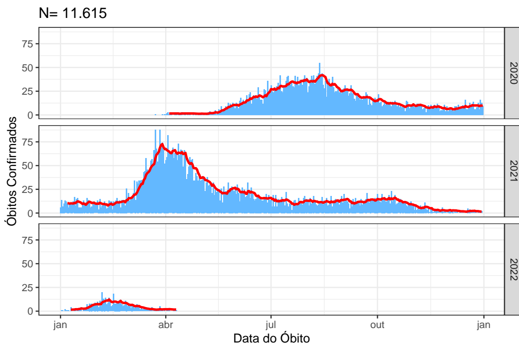
Figura 5: Média móvel dos óbitos confirmados no Distrito Federal, 11 de abril de 2022
