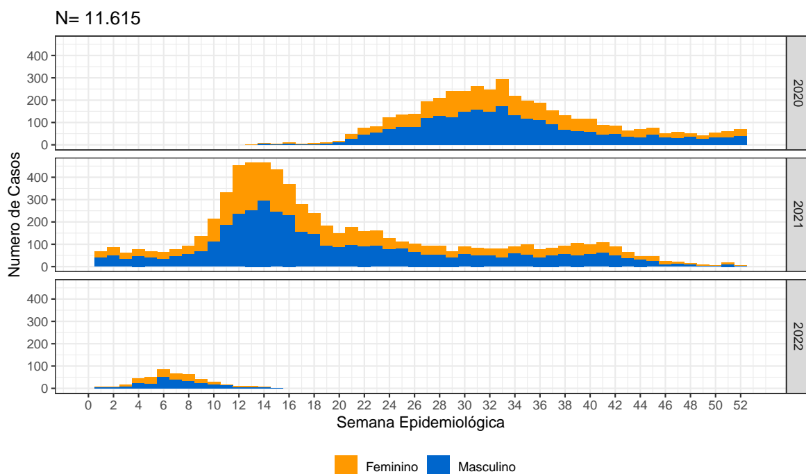
Figura 2: Curva de óbitos confirmados de COVID-19 segundo evolução e data de início de sintomas, Distrito Federal, 11 de abril de 2022
