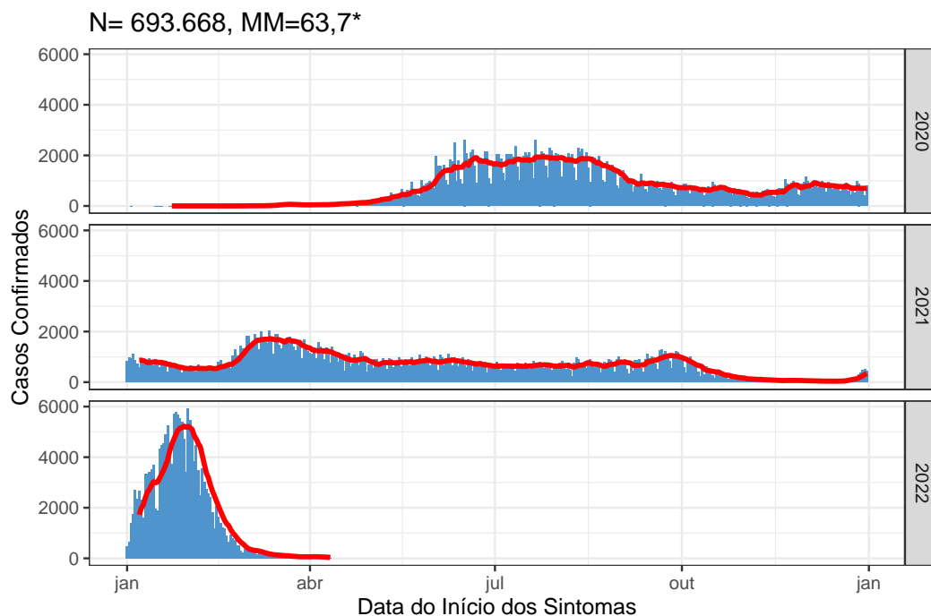
Figura 4: Média móvel dos casos confirmados no Distrito Federal, 11 de abril de 2022
