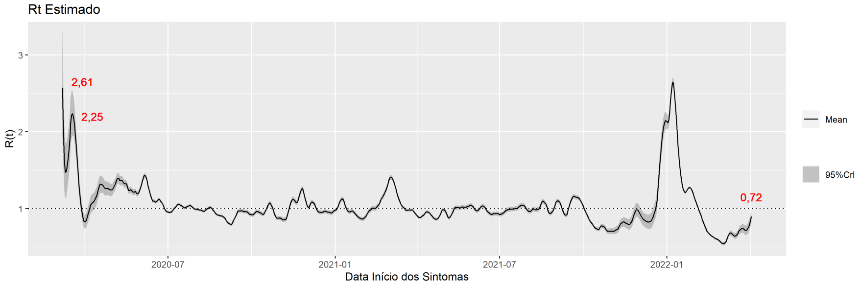
Figura 6: R(t) estimado para os dados oficiais de infectados por Covid-19 no DF segundo a data de início dos sintomas dos casos no Distrito Federal, 11 de abril de 2022
