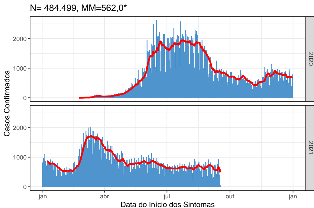
Figura 4: Média móvel dos casos confirmados no Distrito Federal, 18 de setembro de 2021
