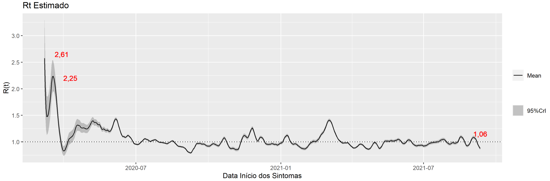
Figura 6: R(t) estimado para os dados oficiais de infectados por Covid-19 no DF segundo a data de início dos sintomas dos casos no Distrito Federal, 18 de setembro de 2021
