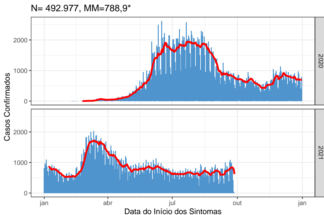
Figura 4: Média móvel dos casos confirmados no Distrito Federal, 27 de setembro de 2021
