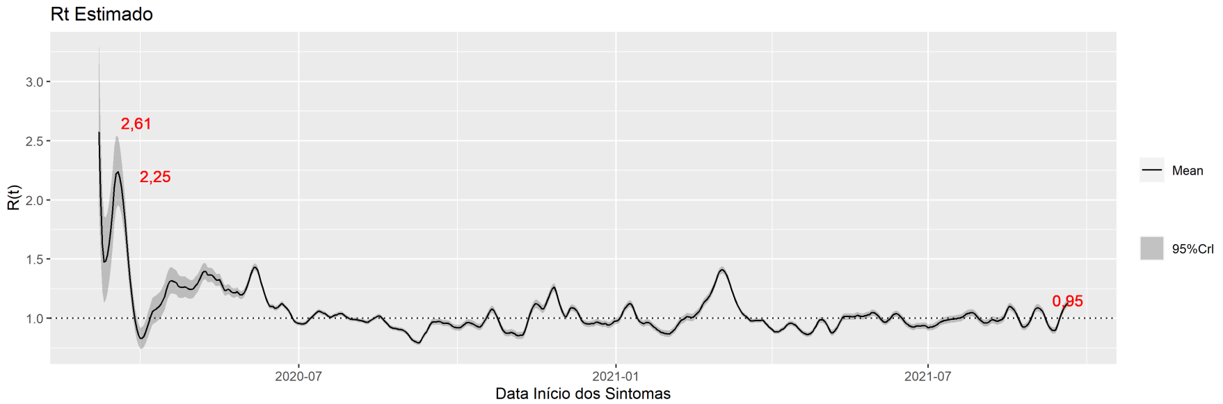
Figura 6: R(t) estimado para os dados oficiais de infectados por Covid-19 no DF segundo a data de início dos sintomas dos casos no Distrito Federal, 27 de setembro de 2021
