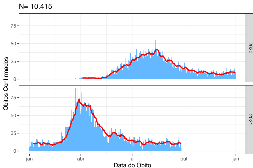
Figura 5: Média móvel dos óbitos confirmados no Distrito Federal, 27 de setembro de 2021
