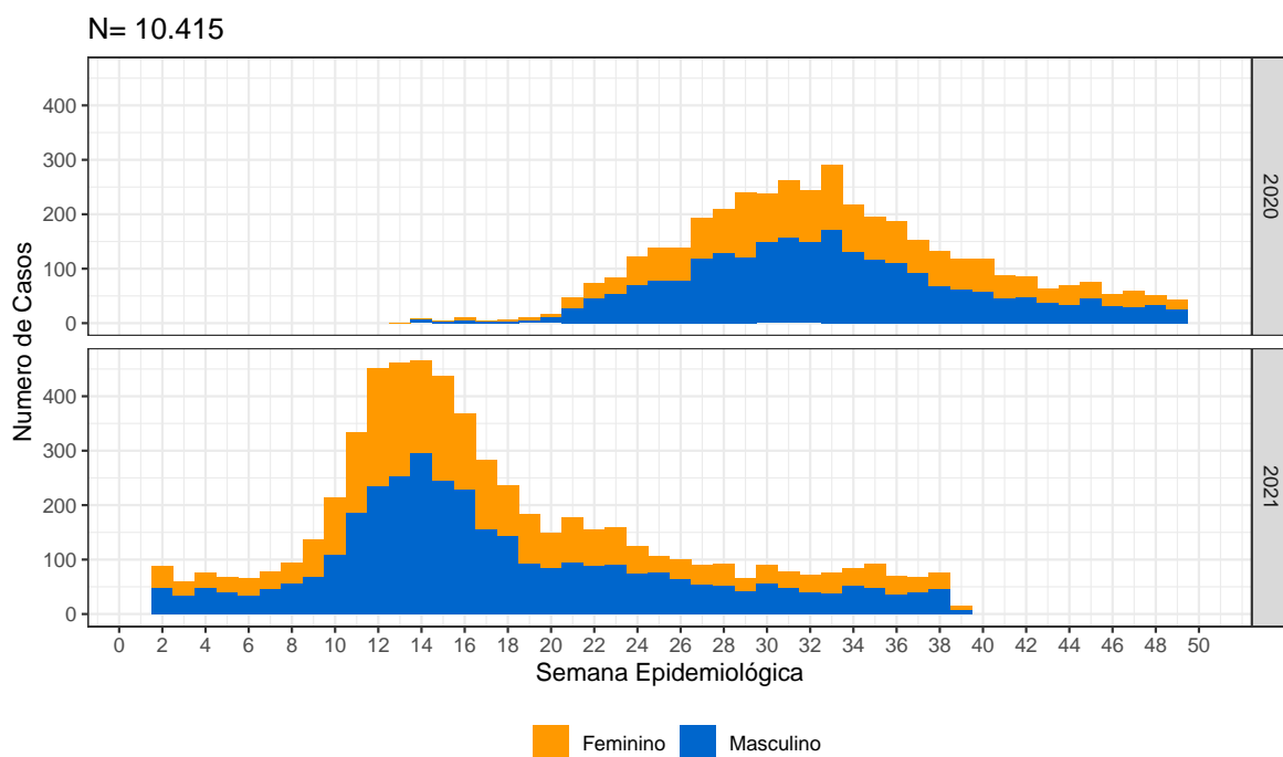
Figura 2: Curva de óbitos confirmados de COVID-19 segundo evolução e data de início de sintomas, Distrito Federal, 27 de setembro de 2021
