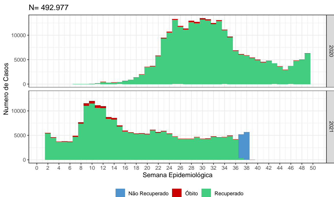
Figura 1: Curva epidemiológica de casos confirmados de COVID-19 segundo evolução e data de início de sintomas, Distrito Federal, 27 de setembro de 2021
