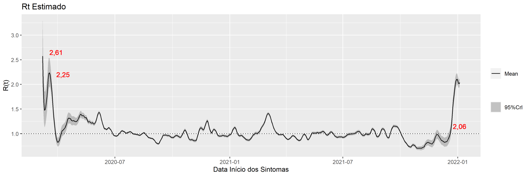
Figura 6: R(t) estimado para os dados oficiais de infectados por Covid-19 no DF segundo a data de início dos sintomas dos casos no Distrito Federal, 11 de janeiro de 2022
