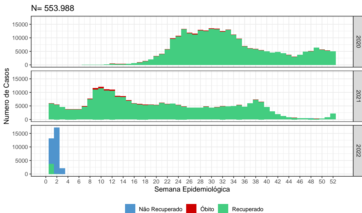
Figura 1: Curva epidemiológica de casos confirmados de COVID-19 segundo evolução e data de início de sintomas, Distrito Federal, 19 de janeiro de 2022
