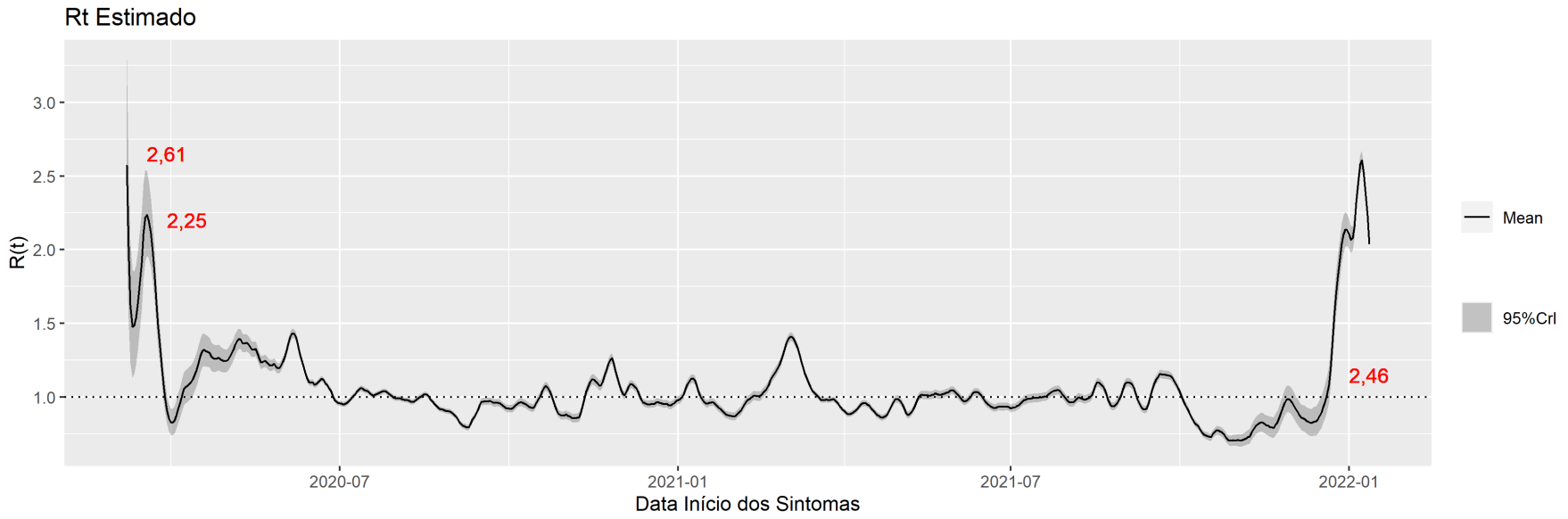
Figura 6: R(t) estimado para os dados oficiais de infectados por Covid-19 no DF segundo a data de início dos sintomas dos casos no Distrito Federal, 19 de janeiro de 2022
