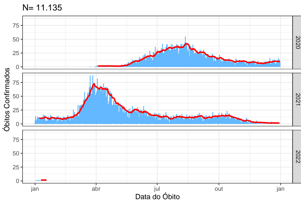
Figura 5: Média móvel dos óbitos confirmados no Distrito Federal, 19 de janeiro de 2022
