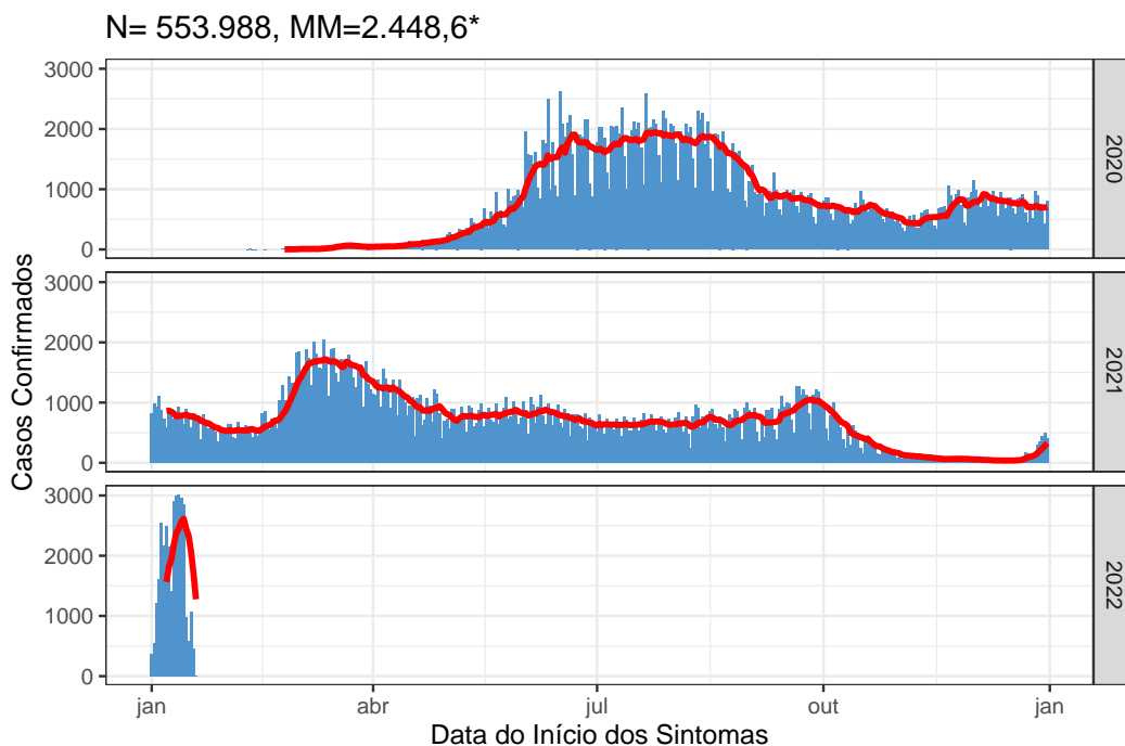
Figura 4: Média móvel dos casos confirmados no Distrito Federal, 19 de janeiro de 2022
