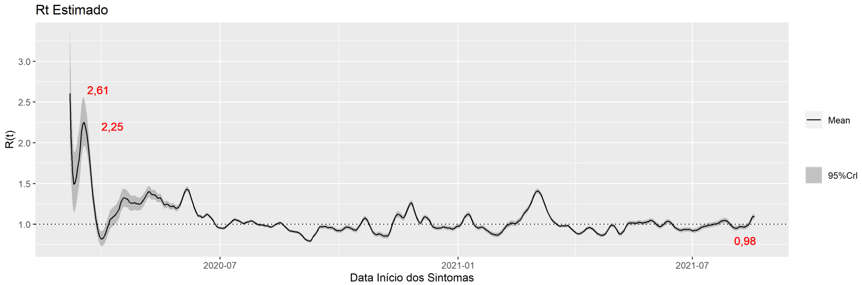
Figura 6: R(t) estimado para os dados oficiais de infectados por Covid-19 no DF segundo a data de início dos sintomas dos casos no Distrito Federal, 25 de agosto de 2021
