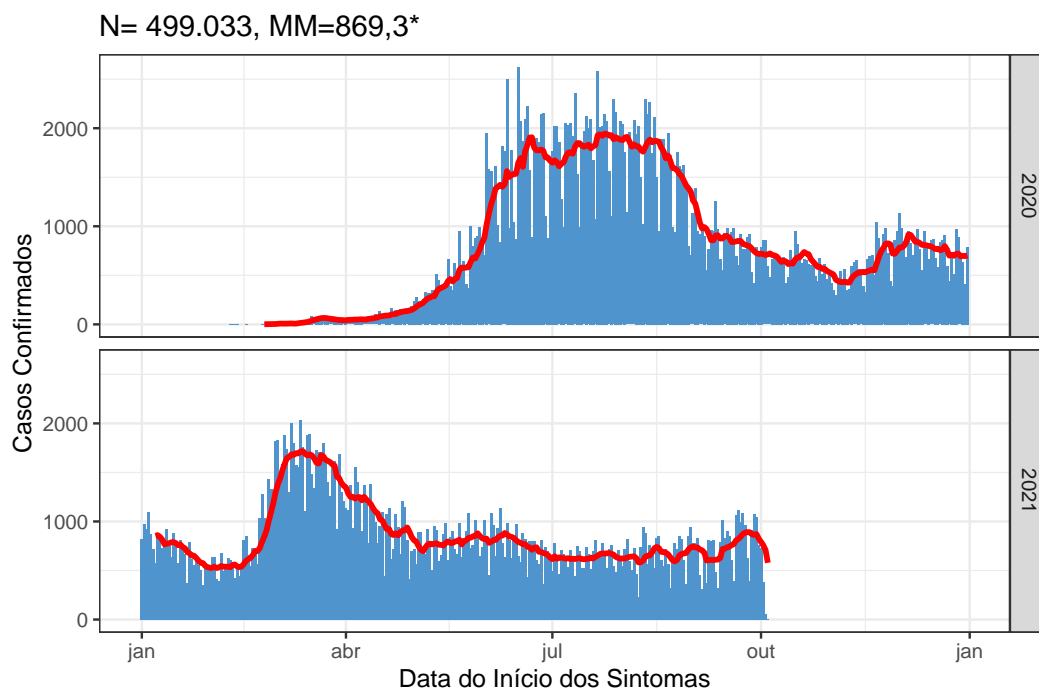
Figura 4: Média móvel dos casos confirmados no Distrito Federal, 04 de outubro de 2021
