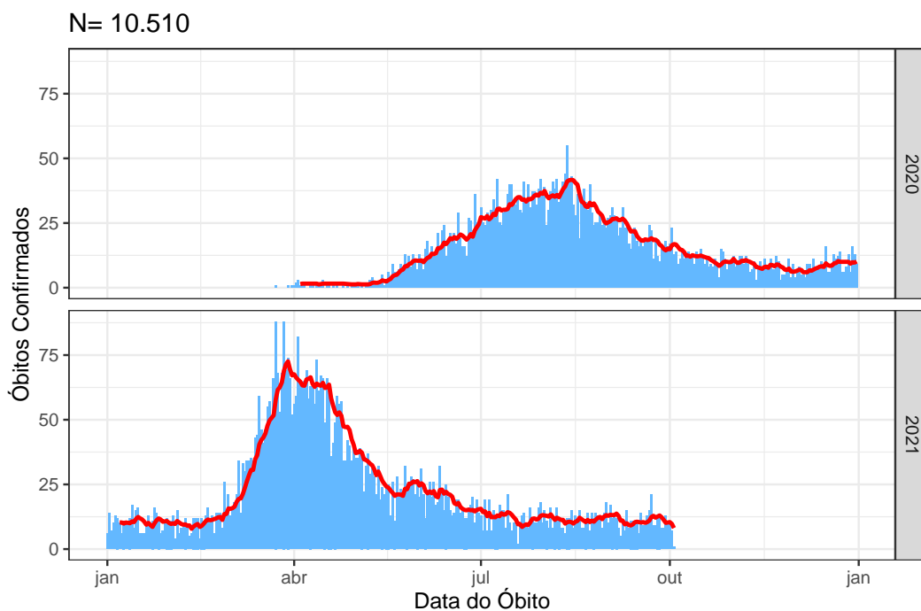
Figura 5: Média móvel dos óbitos confirmados no Distrito Federal, 04 de outubro de 2021
