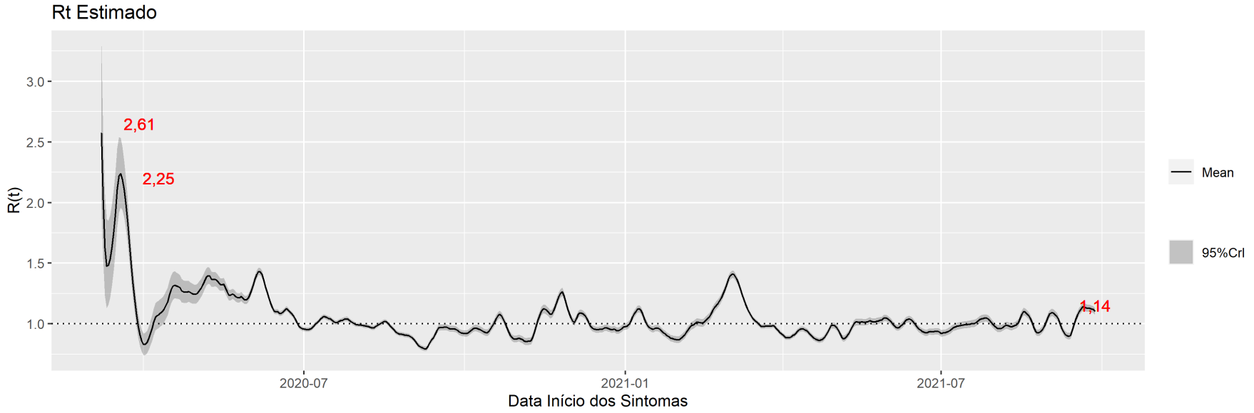
Figura 6: R(t) estimado para os dados oficiais de infectados por Covid-19 no DF segundo a data de início dos sintomas dos casos no Distrito Federal, 04 de outubro de 2021
