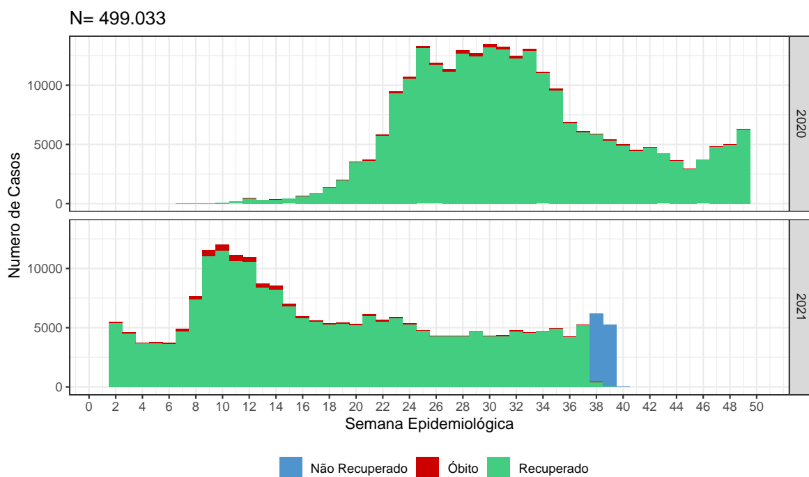
Figura 1: Curva epidemiológica de casos confirmados de COVID-19 segundo evolução e data de início de sintomas, Distrito Federal, 04 de outubro de 2021
